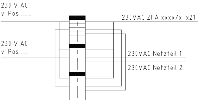
Detail Aufbau Klemmleiste X2
